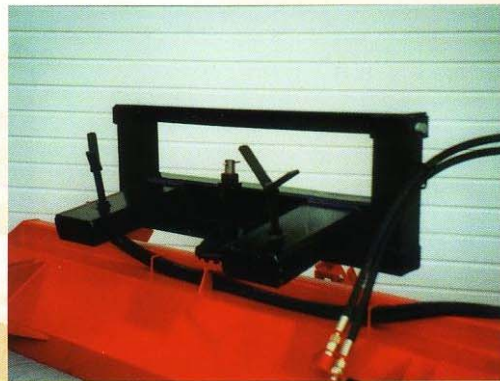
Gabelstapler-Anbau mit Pendelausgleich
