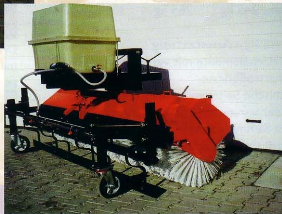
Kehrmaschine mit Kratzer und Sprüheinrichtung
